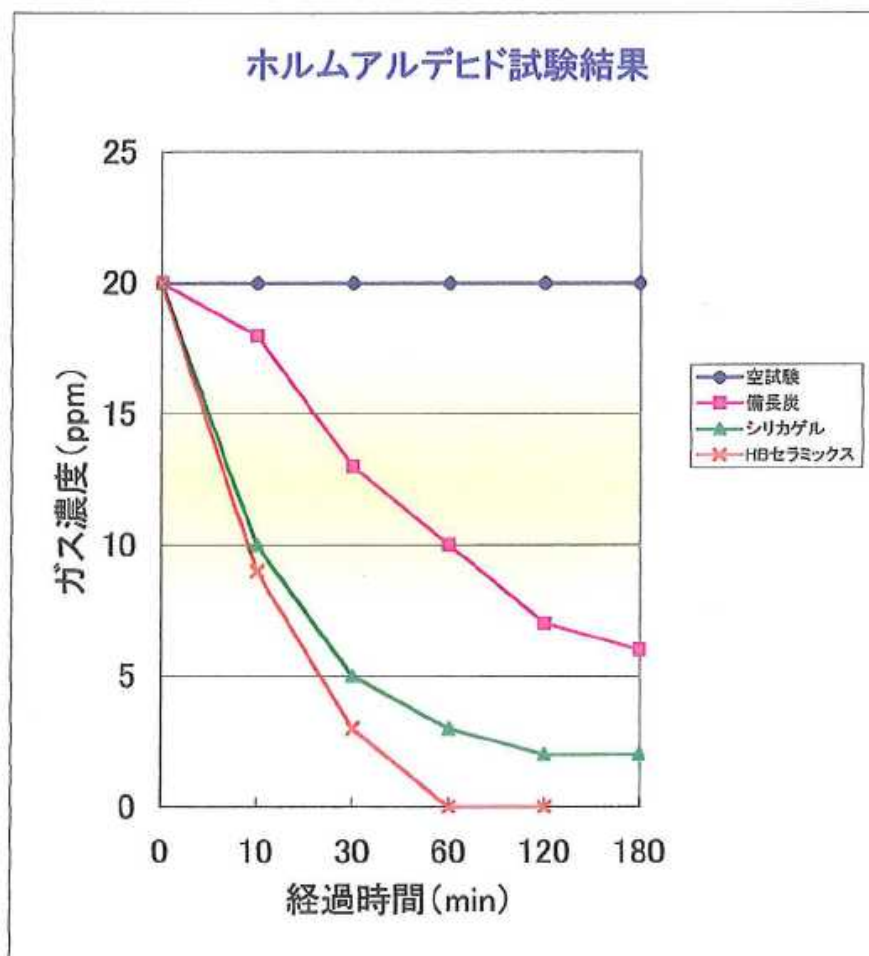
図一2 ホルムアルデヒドの試験結果
