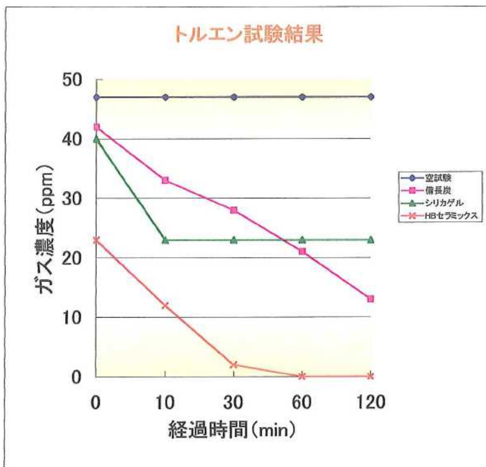
図一トルエンの試験結果
