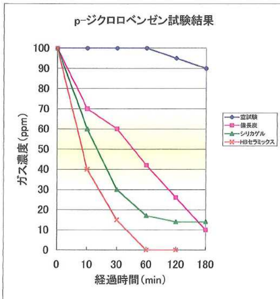
図-3 p-ジクロロベンゼンの試験結果
